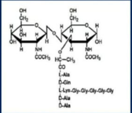
Peptidoglycan
